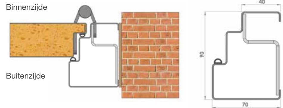
VERSTEKFRAME MET AANSLAG, BINNENDRAAIEND (LI)
